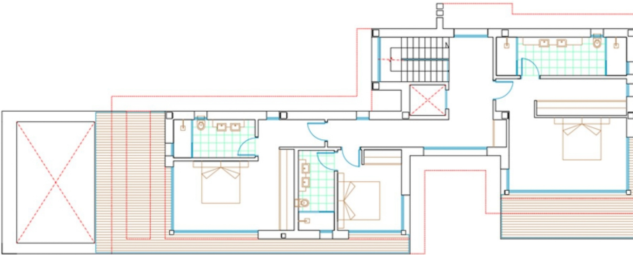
PLANTA PRIMERA
